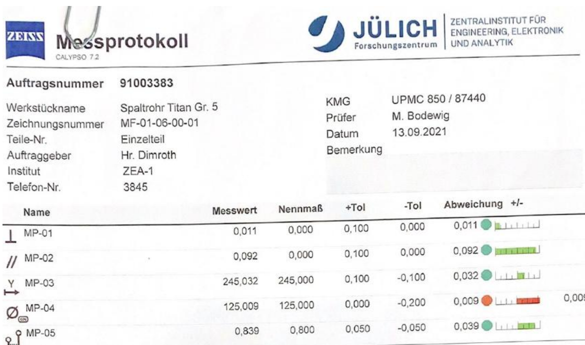
Abbildung C.8: Messprotokoll Spaltrohr
