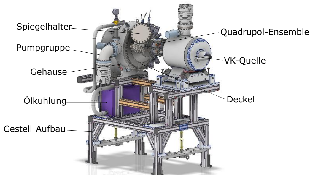
Abbildung 7.9: CAD Modell der Quelle ohne IR-Kamera und Kollimator
