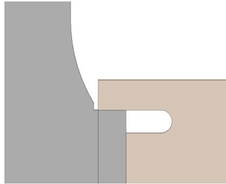
Abbildung 5.6: Radialer Zentriersitz des Targets. Grau: Target. Braun: Kragen des Rotorträger-rechts
