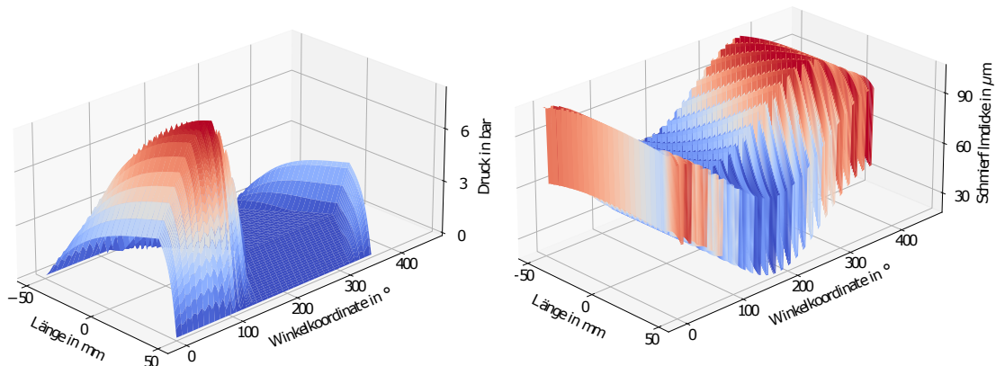
Abbildung 4.20: Links: Druckverteilung der finalen radialen Lagergeometrie unter Berücksichtigung von Kavitationseffekten; rechts: Schmierfilmdicke des Radiallagers
