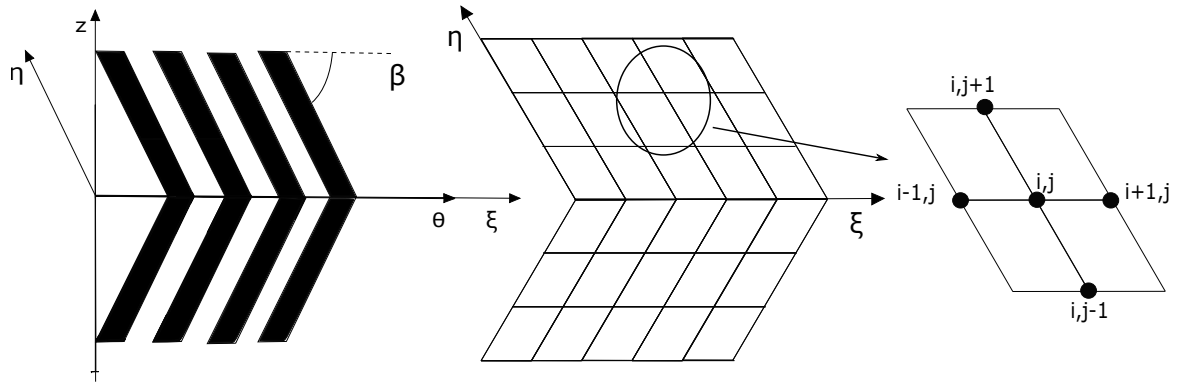
Abbildung 4.10: Links: Transformation kartesischer Koordinaten \theta und z zu schrägen Koordinaten \xi und \eta . Rechts: Darstellung der schrägen Rechendomäne zur Lösung des FDM-Verfahrens
