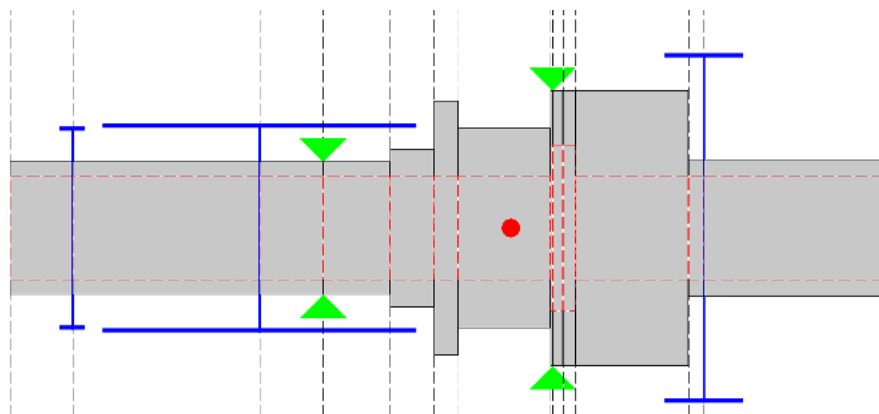
Abbildung 5.20: Modell des Rotors, blau entspricht den Trägheiten, grün den Lagerstellen.
