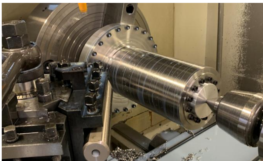
Abbildung 5.19: Spaltrohr in der Endbearbeitungsspannung
