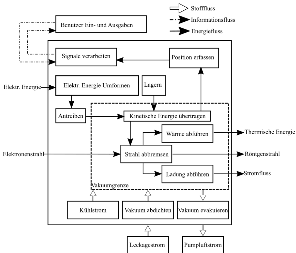
Abbildung 3.2: Funktionsstruktur
