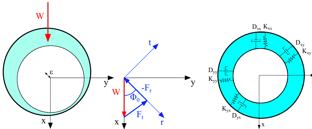
Abbildung 4.5: Links: statische Größen des Lagers mit Tangential- und Radialkraft, störungsbedingter Auslenkung \epsilon und Schwimmwinkel \Phi_0 . Rechts: dynamische Größen des Lagers mit Steifigkeit und Dämpfung
