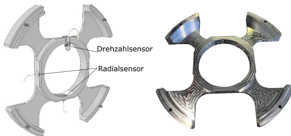
Abbildung 6.8: Links: CAD Darstellung des Sensorhalters. Rechts: Gefertigter Sensorhalter
