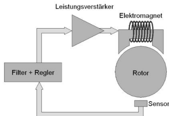
Abbildung 2.2: Funktionsprinzip der aktiven elektromagnetischen Lagerung nach [51]
