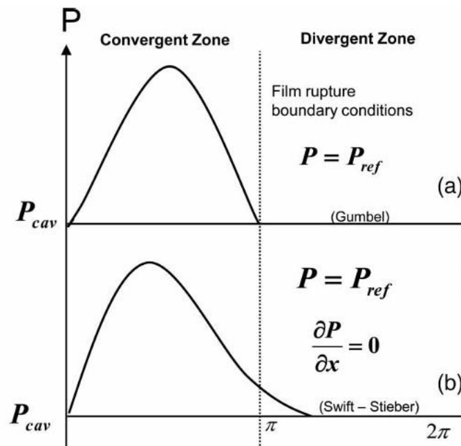
Abbildung 4.4: Kavitationsmodelle aus [23]
