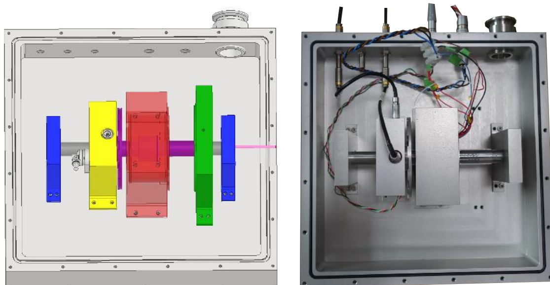
Abbildung 7.1: Links: CAD-Modell Vorversuchsaufbau; Blau: Lagerböcke, Gelb: Sensorhalter, Rot: Stator, Violett: Rotor, Grün: Passives Magnetlager, Pink: Befüllungseinheit. Rechts: Foto des finalen Aufbaus (Deckel nicht dargestellt)
