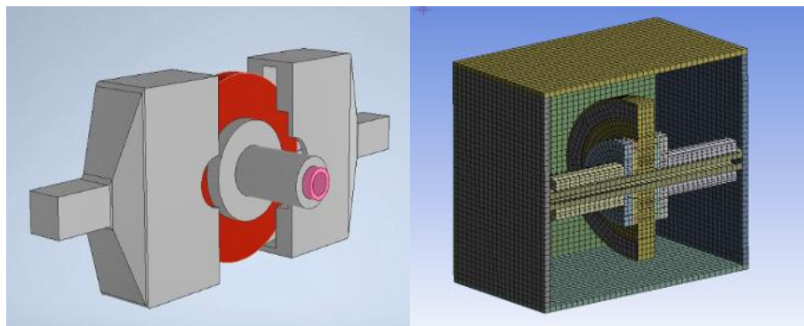
Abbildung 3.4: Links: CAD Modell des Kühlbackenkonzeptes. Rechts: Finite-Elemente-Methode (FEM)-Modell (Netz) mit Außenwänden zur Strahlungsberechnung
