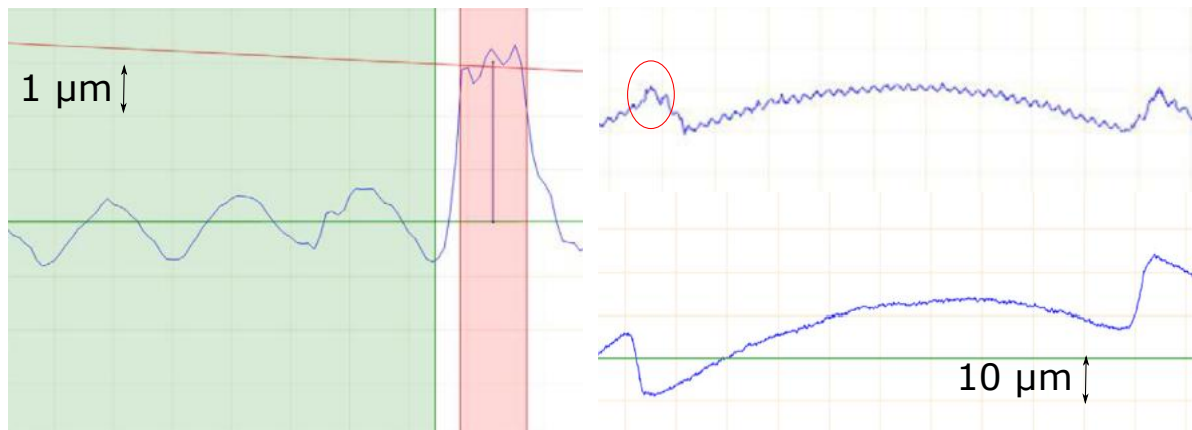
Abbildung 5.22: Auszug aus Weißlichtinterferometrie-Vermessung. Links: Überhöhung in Folge von Materialaufschub beim Fräsen. Rechts oben: Oberfläche nach Fräsbearbeitung, Rechts unten: Oberfläche nach Laserabtrag
