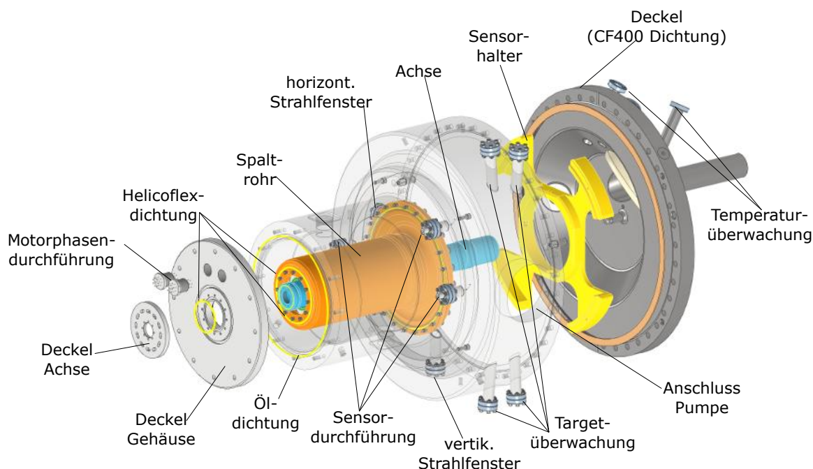
Abbildung 6.5: Explosionsdarstellung der Vakuumkammer. Rotorträger und Target sind nicht dargestellt.
