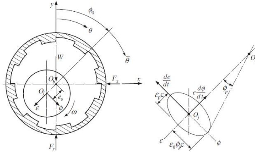
Abbildung 4.6: Wirbelbewegung des Rotors im hydrodynamischen Lager nach [27]; links: statische Gleichgewichtsposition und Schwimmwinkel \phi_0 . Rechts: Störungskordinaten
