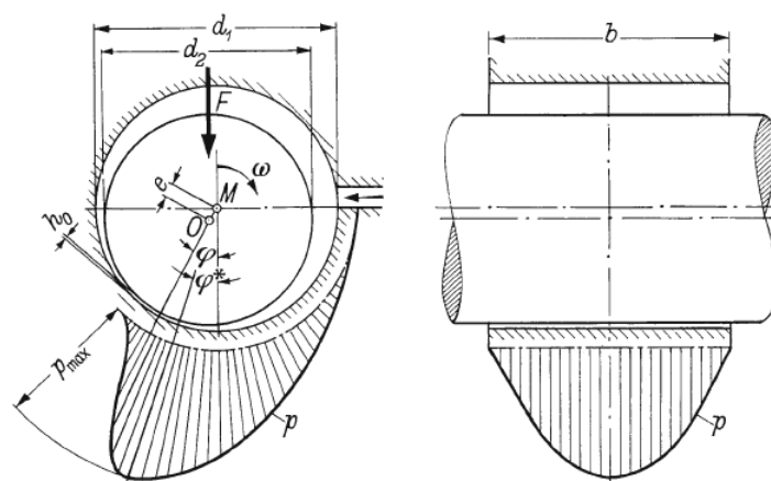
Abbildung 2.3: Schematischer Druckverlauf eines hydrodynamischen Lagers nach [137]
