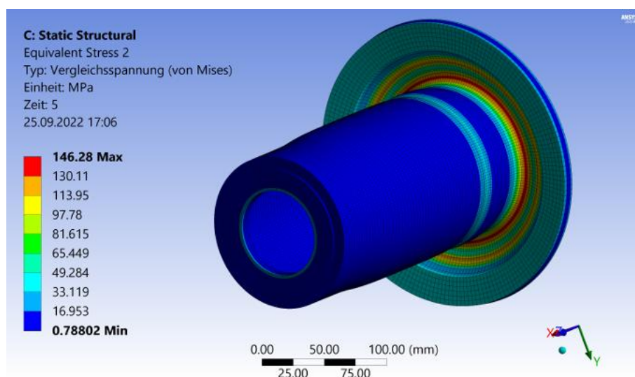
Abbildung 5.18: Spaltrohr unter Temperatur-, Vakuum- und Dehnungslast von -0,2 \text{ MPa}
