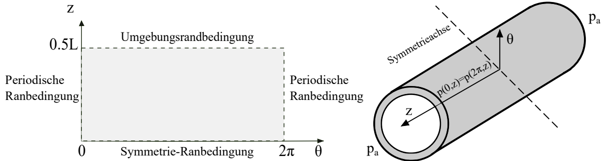
Abbildung 4.3: Randbedingungen für die Anwendung der Reynoldsgleichung (ohne Darstellung des Rillenmusters)
