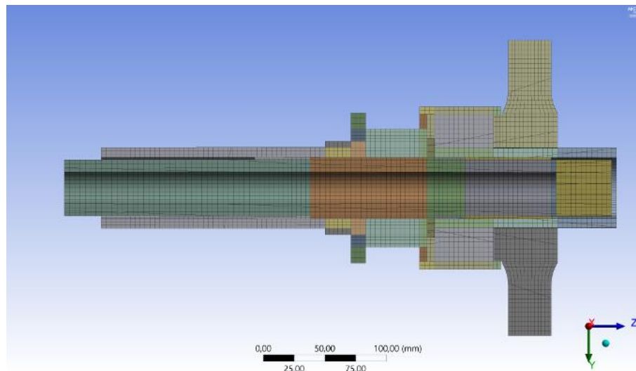
Abbildung 5.10: Hexagonales Netz
