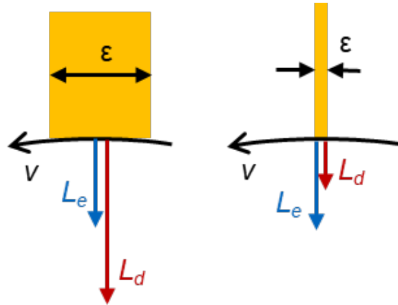
Abbildung 2.10: Links: lange Bestrahlungszeit durch große Brennfleckbreite, große Diffusionslänge und kleiner Elektroneneindringtiefe. Rechts: schmaler Brennfleck, Elektroneneindringtiefe größer als Diffusionslänge nach [8]
