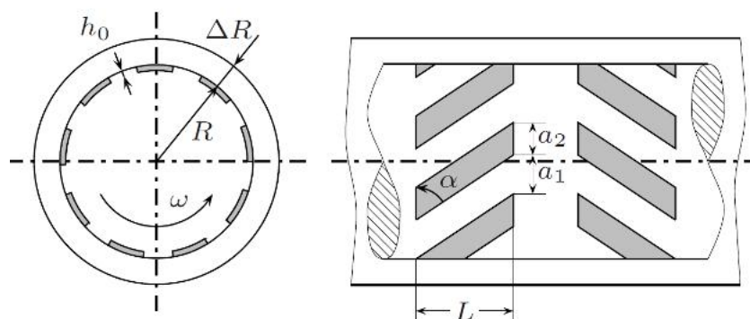
Abbildung 2.4: Prinzipskizze eines Radialrillengleitlagers nach [137]
