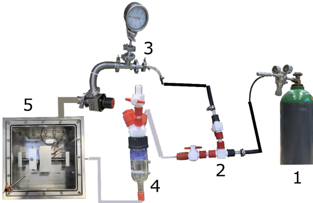
Abbildung 7.5: Befüllungsaufbau bestehend aus 1 Argongasflasche, 2 T-Stück mit Kugelhähnen, 3 Druckmessgerät mit Ventil, 4 Glasgefäß mit Kugelhahn und 5 Aufbau
