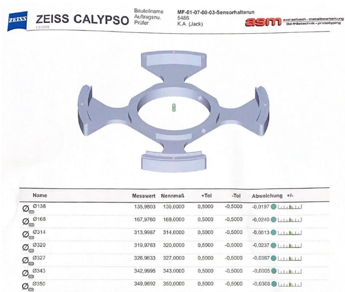
Abbildung C.7: Messprotokoll Sensorhalter
