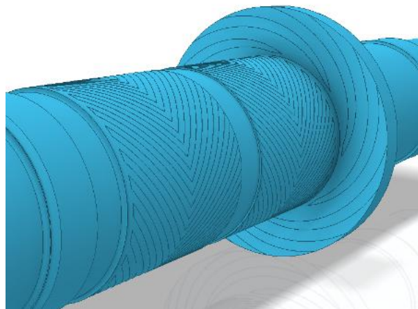
Abbildung 4.1: CAD-Modell eines Spiralrillengleitlagers (radial und axial)
