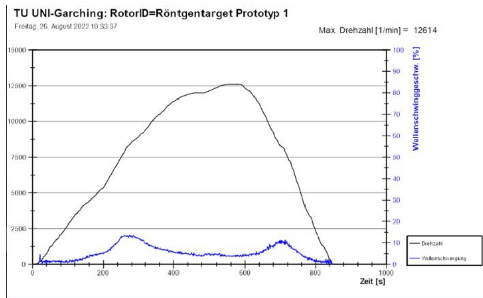
Abbildung C.10: Schleuderversuchsprotokoll Rotorträger-rechts mit Target
