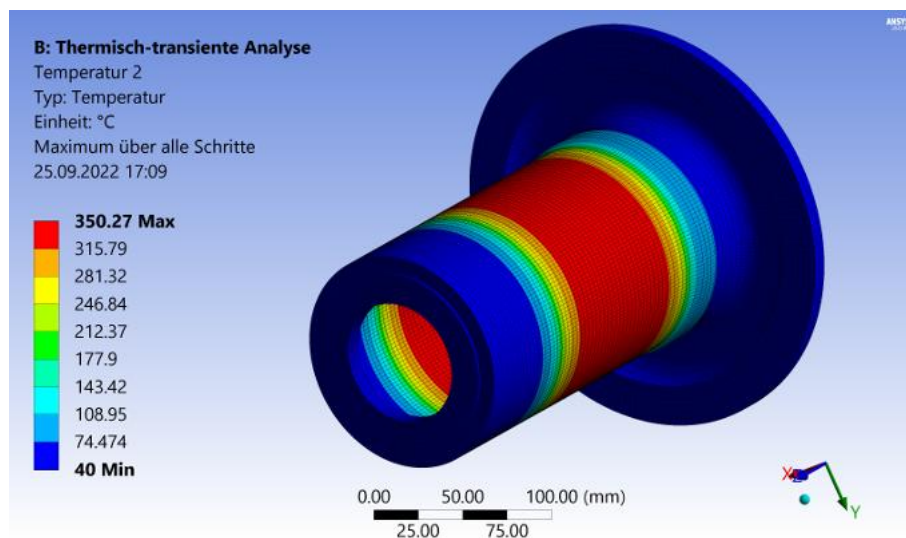
Abbildung 5.17: Maximaler Temperaturanstieg bei minimalem Wärmeübergangskoeffizienten
