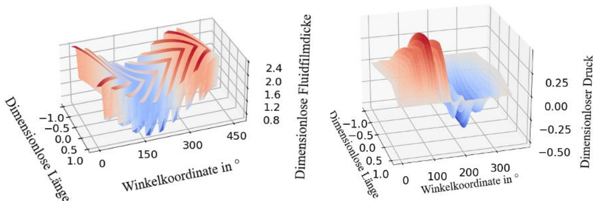
Abbildung 4.15: Links: Schmierfilmdarstellung (dimensionslos) in transformierten Koordinaten. Rechts: Druckverteilung mit Sägezahnverlauf nach lokaler Integrationsmethode
