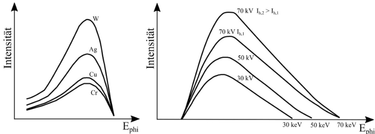
Abbildung 1.1: Intensität über Photonenenergie E_{\text{phi}} ; Links: Schematische Darstellung des Energiespektrums für verschiedene Anodenmaterialien bei konstanter Beschleunigungsspannung und Anodenstrom.
