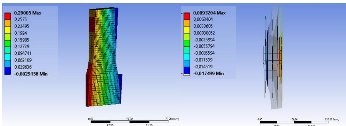
Abbildung 5.8: Links: axiale thermische Dehnung; Rechts: axiale Dehnung durch Rotation
