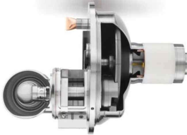
Abbildung 2.7: Seitenansicht von Philips iMRC ® (2007) unter Verwendung von Flüssigmetall geschmierten Radialrillengleitlagern [11]
