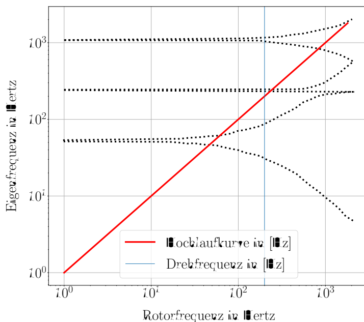
Abbildung 5.21: Numerisch berechnetes Campbell-Diagramm
