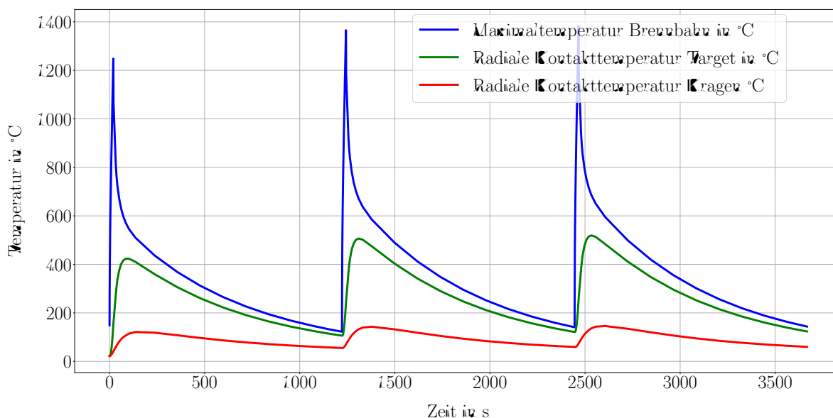
Abbildung 5.12: Temperaturverteilung
