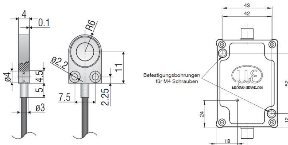
Abbildung 6.7: Links: Schematische Darstellung des Drehzahlsensors. Rechts: Controller zur Pulserfassung und Drehzahlberechnung [98]
