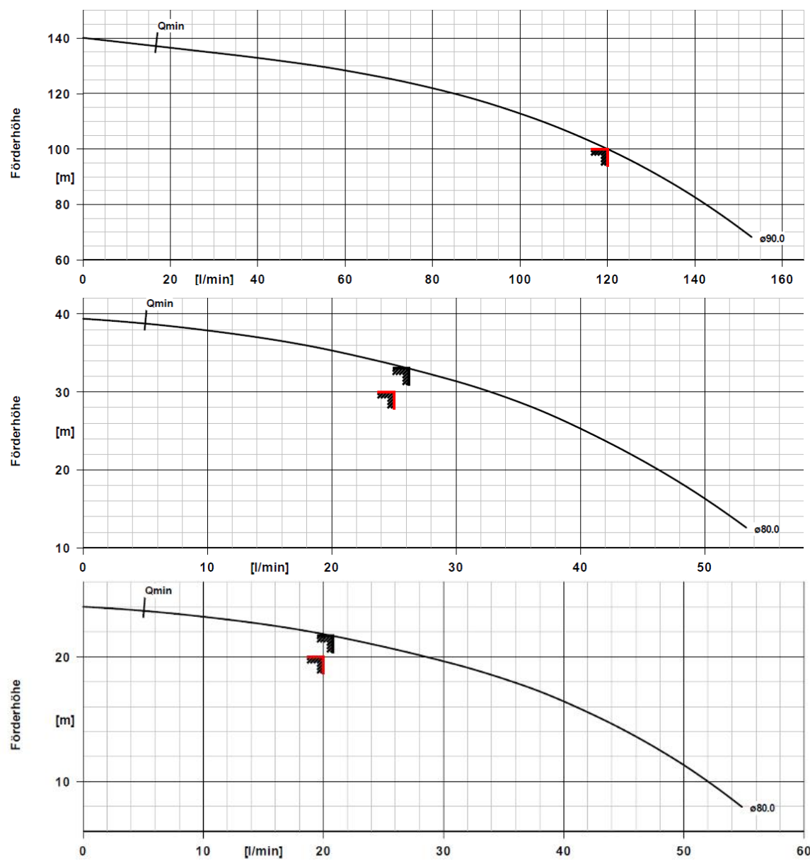
Abbildung D.1: Kennlinien der Pumpen, oben große Pumpe, mittig mittlere Pumpe, unten kleine Pumpe.
