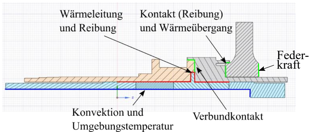
Abbildung 5.11: Überblick wichtigster Randbedingungen (ohne axiale Fixierung)
