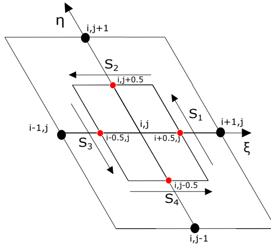
Abbildung 4.13: Integrationsfläche
