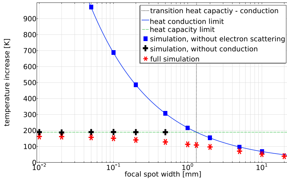
Abbildung 2.11: Maximale Temperaturerhöhung im Brennfleck in der Wärmekapazitätsgrenze (schmaler Brennfleck) und der Wärmeleitungsgrenze (breiter Brennfleck), mit Elektronenstrahlleistung von 90 kW, Energie von 300 keV und Oberflächengeschwindigkeit von 200 m s -1 nach [162]
