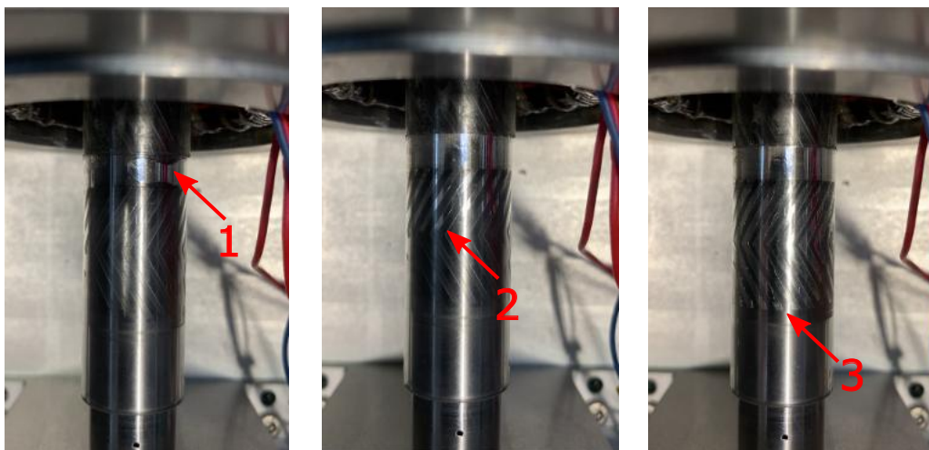
Abbildung 7.6: Fortschritt der Befüllung 1) Austreten der Flüssigkeit aus Bohrung 2) Halbe Befüllung des Lagers 3) Befüllungsverlauf entlang der Fischgrätenstruktur
