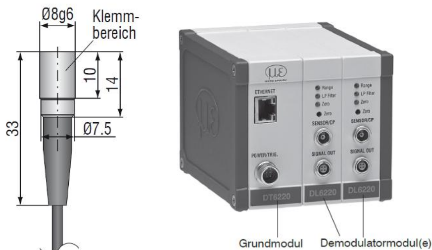
Abbildung 6.6: Links: Schematische Darstellung des Radialsensors Rechts: Controller zur Abstandserfassung [98]
