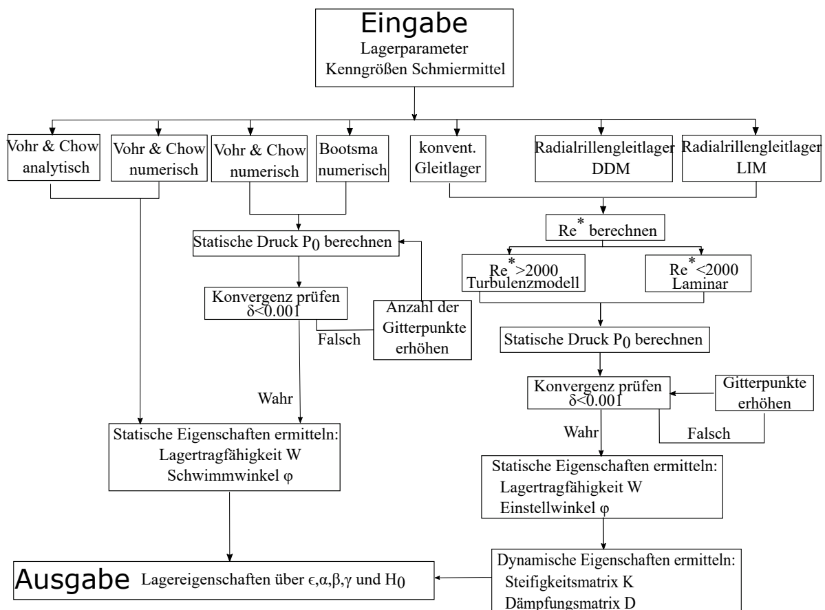
Abbildung 4.14: Programmstruktur
