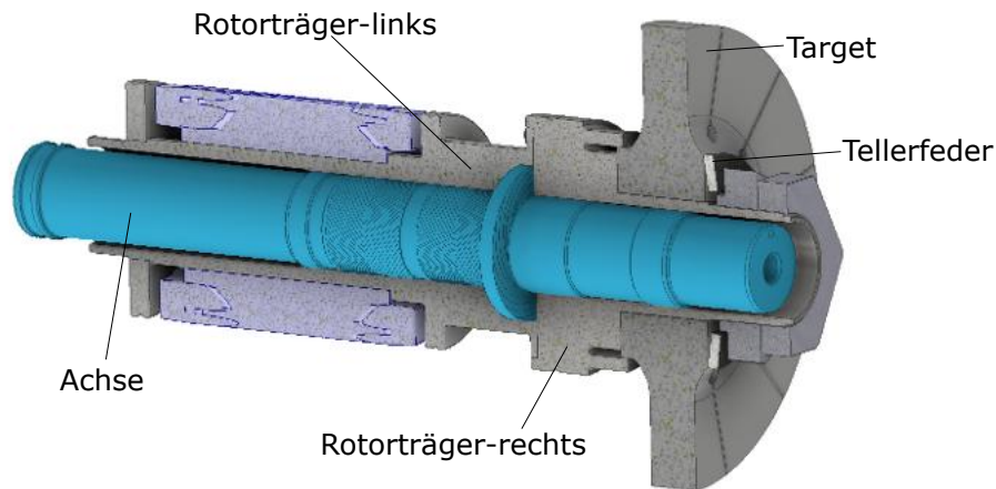
Abbildung 5.1: Rotorbaugruppe bestehend aus Achse, zwei Rotorträgern, Target und Tellerfeder
