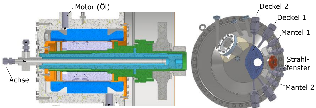
Abbildung 6.3: Rezipienten der Kühlung. Links: Achskühlung und Motorkühlung (Öl). Rechts: Deckelkühlung mit 2 Hauptkreisläufen, 2 Mantelkühlungen und Strahlfensterkühlung
