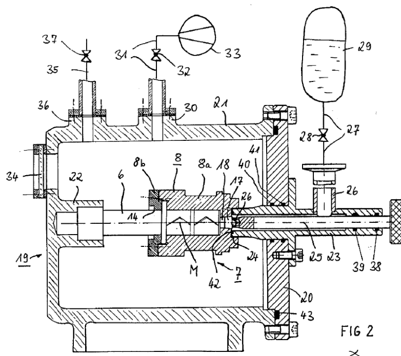
Abbildung 7.4: Prinzipskizze zur Befüllung Flüssigmetall-geschmierter-Gleitlager nach [55]. Positionsbilder werden vernachlässigt.
