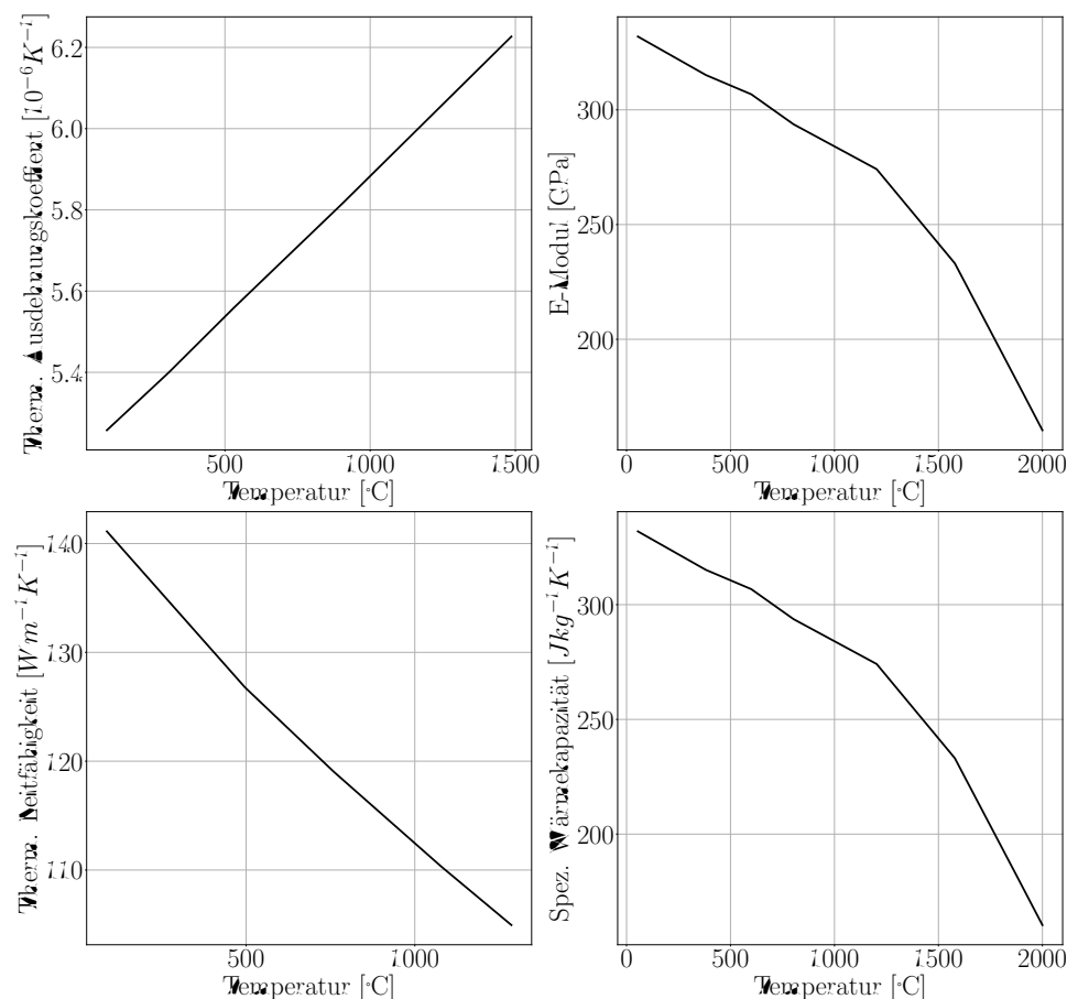
Abbildung 5.4: Werkstoffeigenschaften von TZM in Abhängigkeit der Temperatur nach [94]
