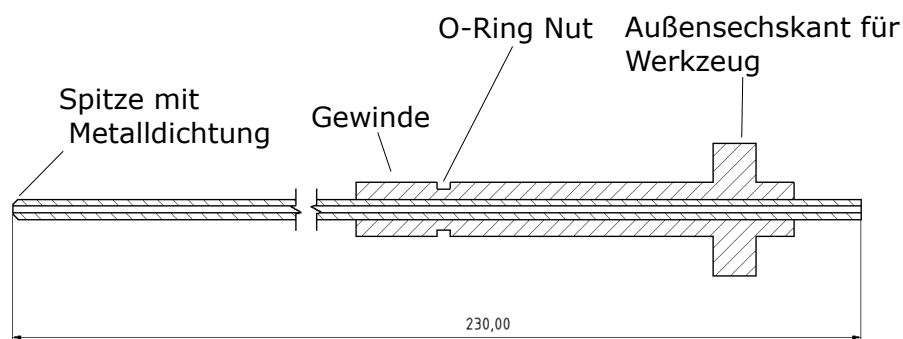
Abbildung 7.7: Skizze der Befüllungshilfe für den finalen Prototypen (Teflonschlauch und O-Ring nicht dargestellt)
