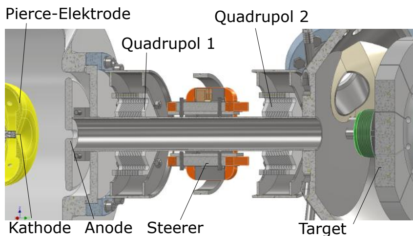
Abbildung 7.10: CAD Modell der Beschleunigerstrecke nach [93]
