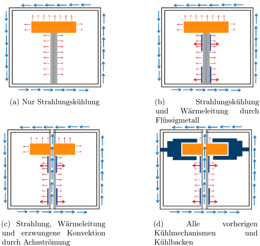
Abbildung 3.3: Vier verschiedene Kühlszenarien der Vorstudie zur Konzeptbestimmung. Umlaufende blaue Pfeile zeigen Umgebungskühlung (freie Konvektion)
