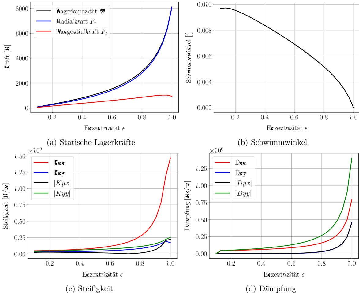
Abbildung 4.21: Finale statische und dynamische Eigenschaften des radialen Lagers
