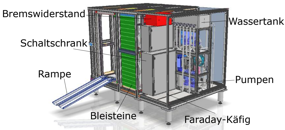
Abbildung 7.13: CAD Modell des Strahlenschutzkabinetts
