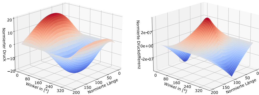
Abbildung 4.9: Links: normierte Druckverteilung nach analytischer Lösung; rechts: Differenz zwischen analytischer und numerischer Lösung nach Gleichung 4.60
