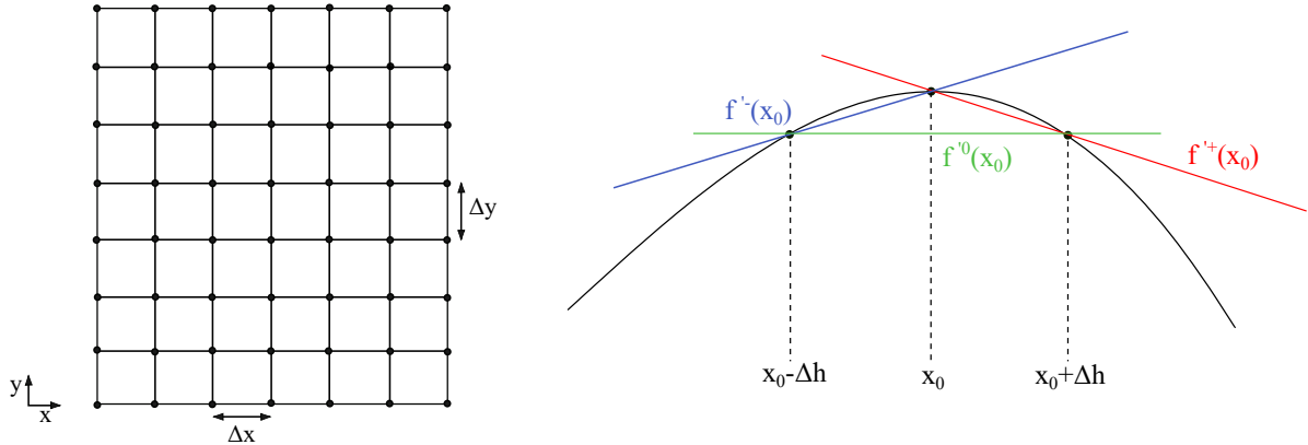
Abbildung 4.8: links: Rechengitter mit Schrittweite \Delta x und \Delta y (zweidimensional); rechts: Differenzenquotienten (eindimensional)
