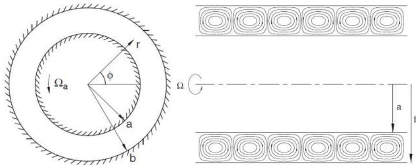
Abbildung 4.24: Darstellung toroidaler Taylorwirbel bei Überschreiten einer kritischen Drehzahl nach [145]
