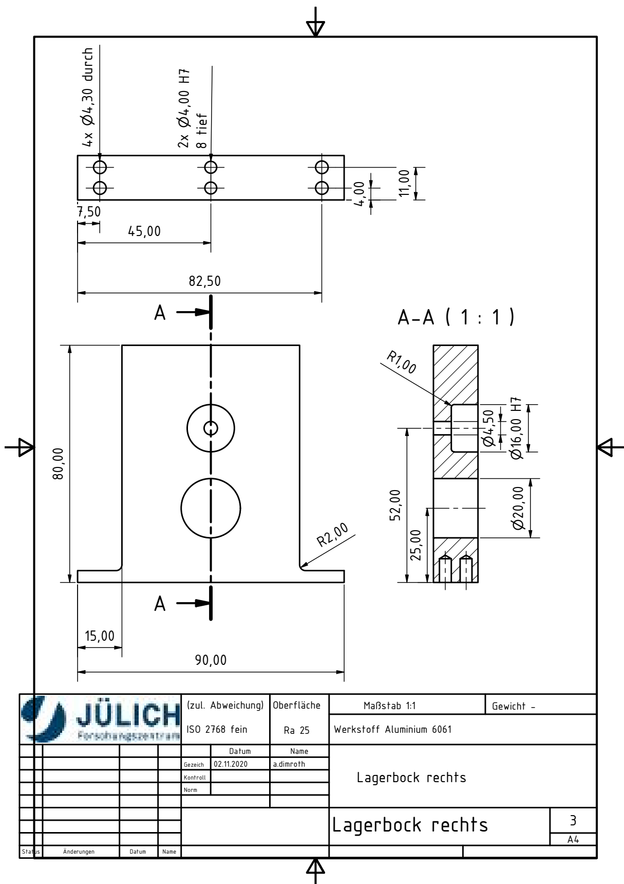
Abbildung B.24: Rechter Lagerbock
