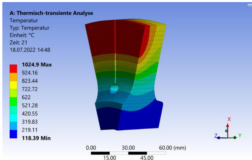
Abbildung 5.3: FEM-Modell des Targets mit hexagonalem Gitter und Wärmeverteilung
