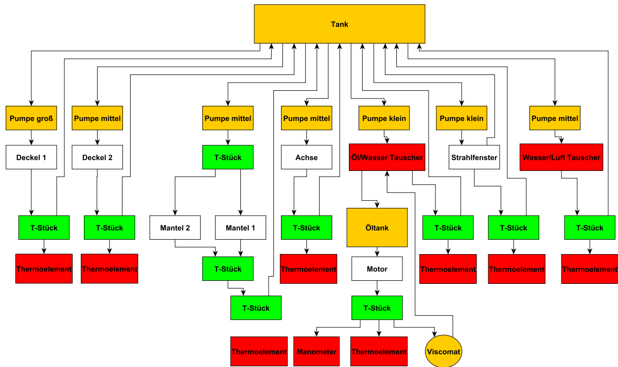
Abbildung 6.4: Flussplan der Kühlkreisläufe
