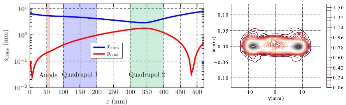
Abbildung 7.11: links: Brennfleckdimensionen der Länge (x) und Breite (y); rechts: Normierte Elektronenintensität des Brennflecks nach [93]
