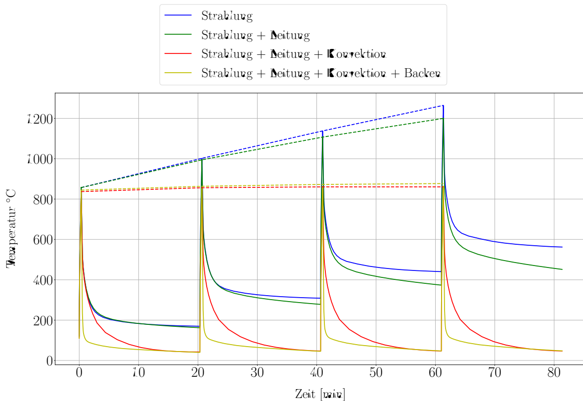
Abbildung 3.5: Maximale Brennbahntemperatur nach vier Bestrahlungszyklen nach [162]
