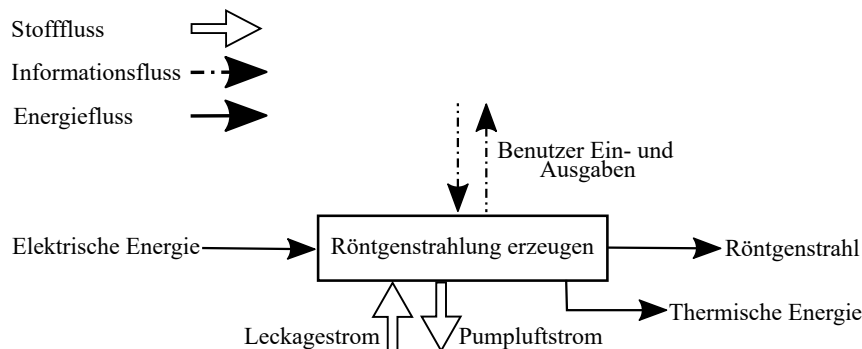
Abbildung 3.1: Schematische Darstellung der Gesamtfunktion einer Röntgenröhre
