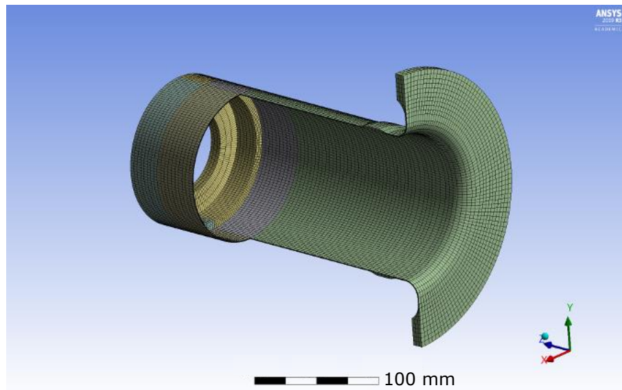
Abbildung 5.16: Halbschnittsdarstellung des hexagonalen Netzes des Spaltrohres
