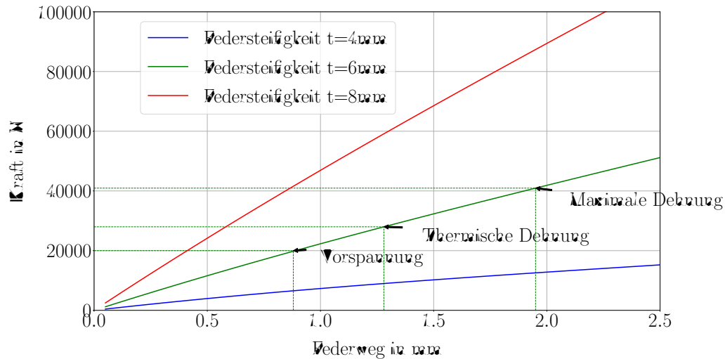
Abbildung 5.9: Federkennlinie
