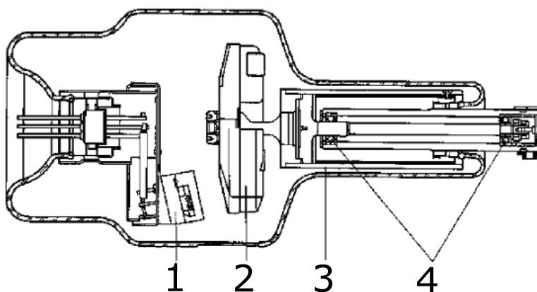
Abbildung 2.6: Konventionelle Drehanodenröhre mit 1)Kathode 2)Drehanode 3)Rotor 4)Kugellager nach [122]
