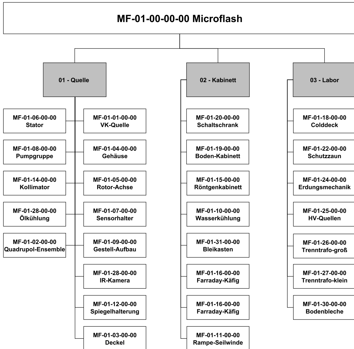
Abbildung 7.8: Einteilung des Gesamtsystems in Module und Baugruppen
