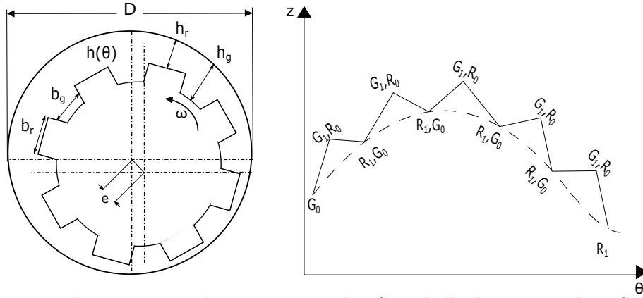
Abbildung 4.7: Links: geometrische Parameter des Sprialrillenlagers. Rechts: Sägezahn- und geglättete Druckverteilung nach [153]
