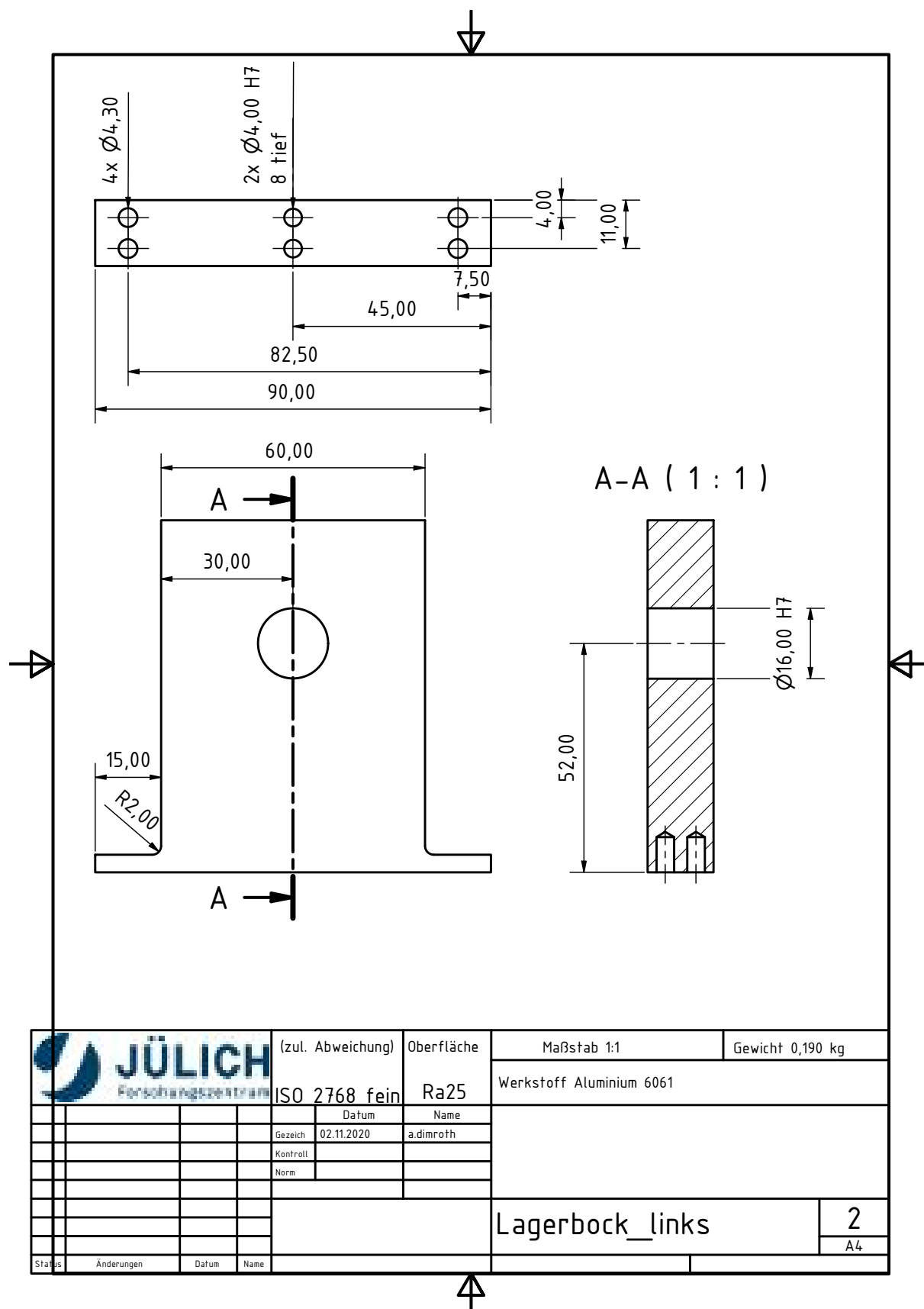
Abbildung B.23: Linker Lagerbock
