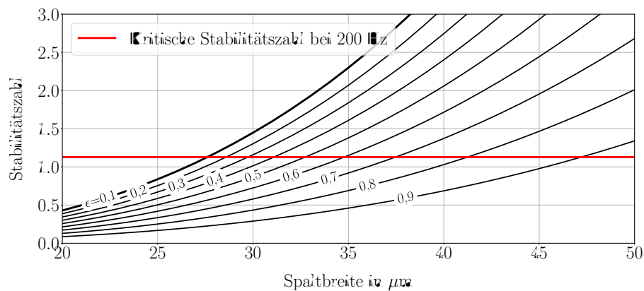
Abbildung 4.19: Stabilitätszustände des Lagers in Abhängigkeit der konzentrischen Spaltbreite ( C, \Delta R ) bei verschiedenen Exzentrizitäten \epsilon für eine Drehzahl von 200 U/min
