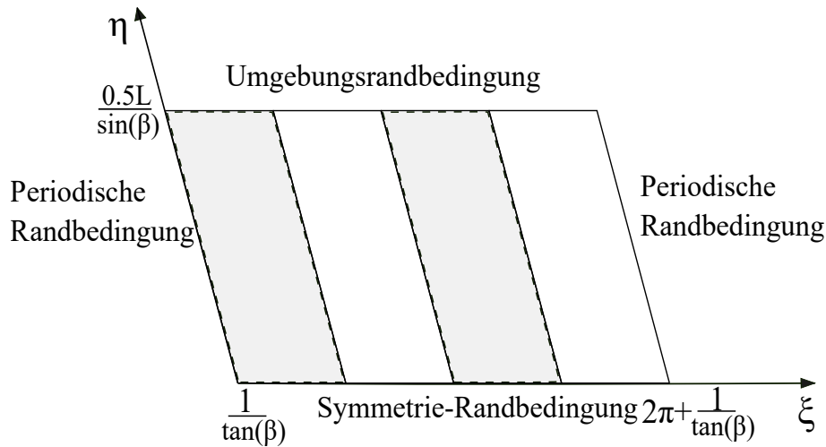
Abbildung 4.12: Randbedingungen im schrägen Koordinatensystem
