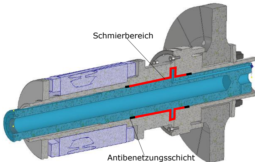
Abbildung 5.23: Schnittdarstellung des Antriebstrangs mit Kennzeichnung der Benetzungsschicht (rot) und der Antibenetzungsschicht (schwarz)
