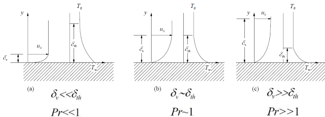
Abbildung 4.22: Einfluss der Prandtlzahl auf die viskose und thermische Grenzschicht bei konstanter Wandtemperatur nach [44]
