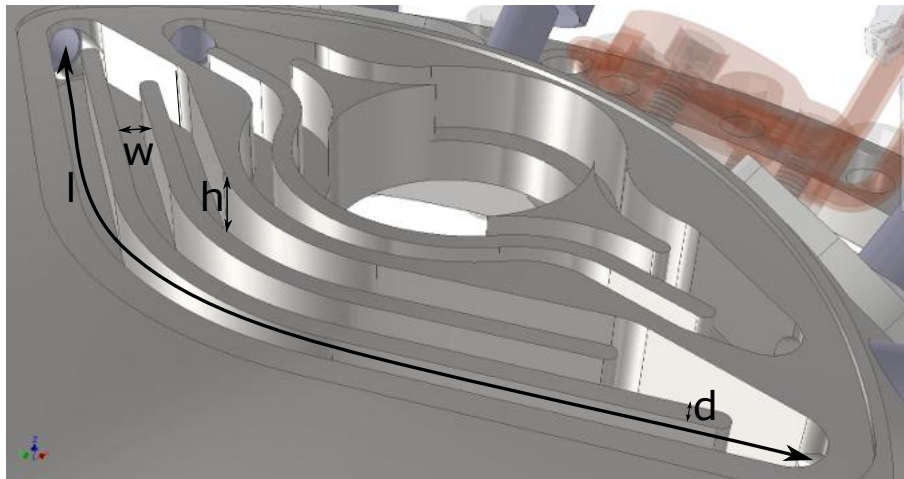
Abbildung 6.2: CAD Modell der Rippengeometrie mit l als Kanallänge, w als Kanalbreite, h als Kanalhöhe und d als Rippenbreite
