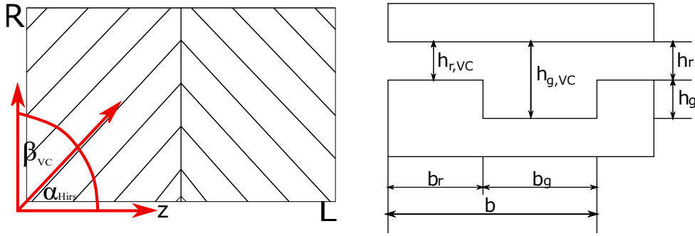
Abbildung 4.2: Parameter zur Beschreibung des Spiralrillengleitlagers; links: Fischgrätenmuster mit radialer Richtung R , und Längsrichtung z ; rechts: Darstellung eines Rille-Damm-Paares
