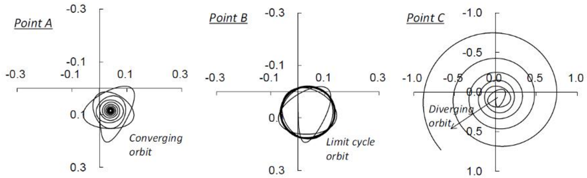
Abbildung 4.18: Stabilitätszustände des Lagers; links: konvergierender Orbit (stabil). Mitte: konstanter Orbit (noch stabil). Rechts: divergierender Orbit (instabil) nach [101]
