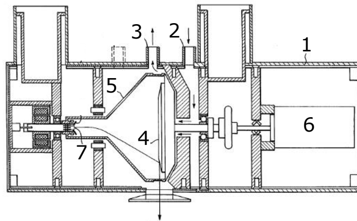
Abbildung 2.9: Drehkolbenröhre mit Direktkühlung [122]. Gehäuse (1); Ölzufuhr (2); Ölabfuhr (3); Drehanode (4); Vakuumkammer (5); Motor (6); Kathode(7)
