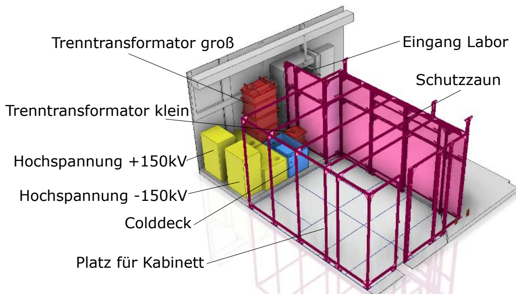
Abbildung 7.12: CAD Modell des Raumes ohne Kabinett Im Labor ist ein Schutzzaun vorgesehen, der das Kabinett umschließt und so den Bereich der Hochspannung absichert. Mit einer Gesamtbeschleunigungsspannung von 300\text{ kV} werden zwei
