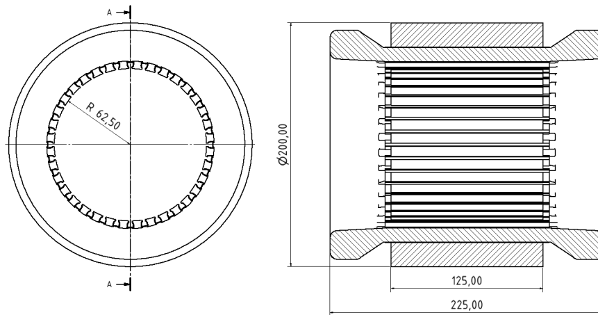
Abbildung 5.15: Technische Skizze der Statorabmessungen
