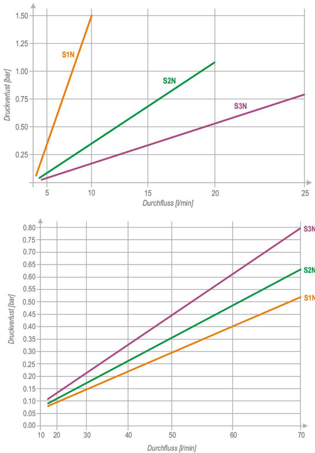
Abbildung D.2: Kennlinien Ölwärmetauscher; oben: Kreislauf B; unten: Kreislauf A
