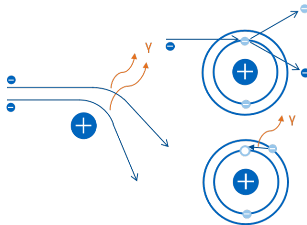
Abbildung 1.2: links: Bremsstrahlung, rechts: charakteristische Strahlung nach [124]
