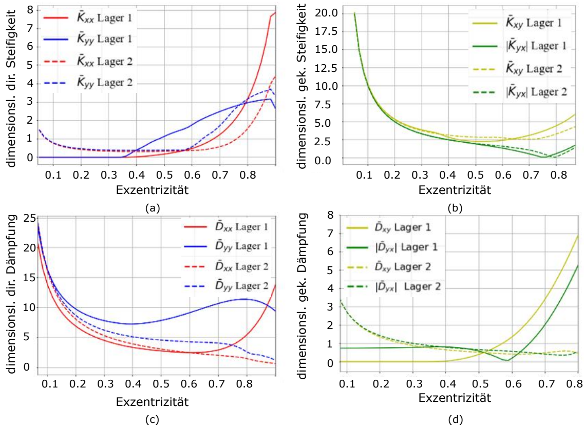
Abbildung 4.17: Gegenüberstellung dynamischer Lagereigenschaften von konventionellem Gleitlager (Lager 1) und Hirs Beispiellager (Lager 2) (a) direkte Steifigkeitskoeffizienten; (b) gekoppelte Steifigkeitskoeffizienten (c) direkte Dämpfungskoeffizienten; (d) gekoppelte Dämpfungskoeffizienten
