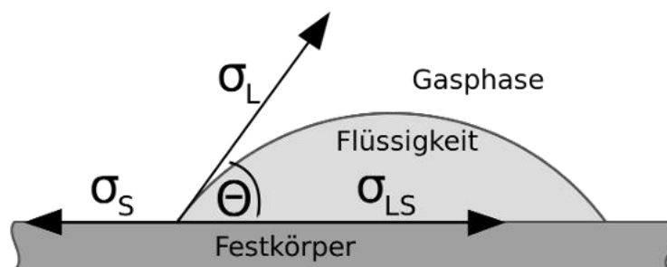
Abbildung 5.24: Schematische Darstellung des Kontaktwinkels bei einem liegenden Tropfen [57]
