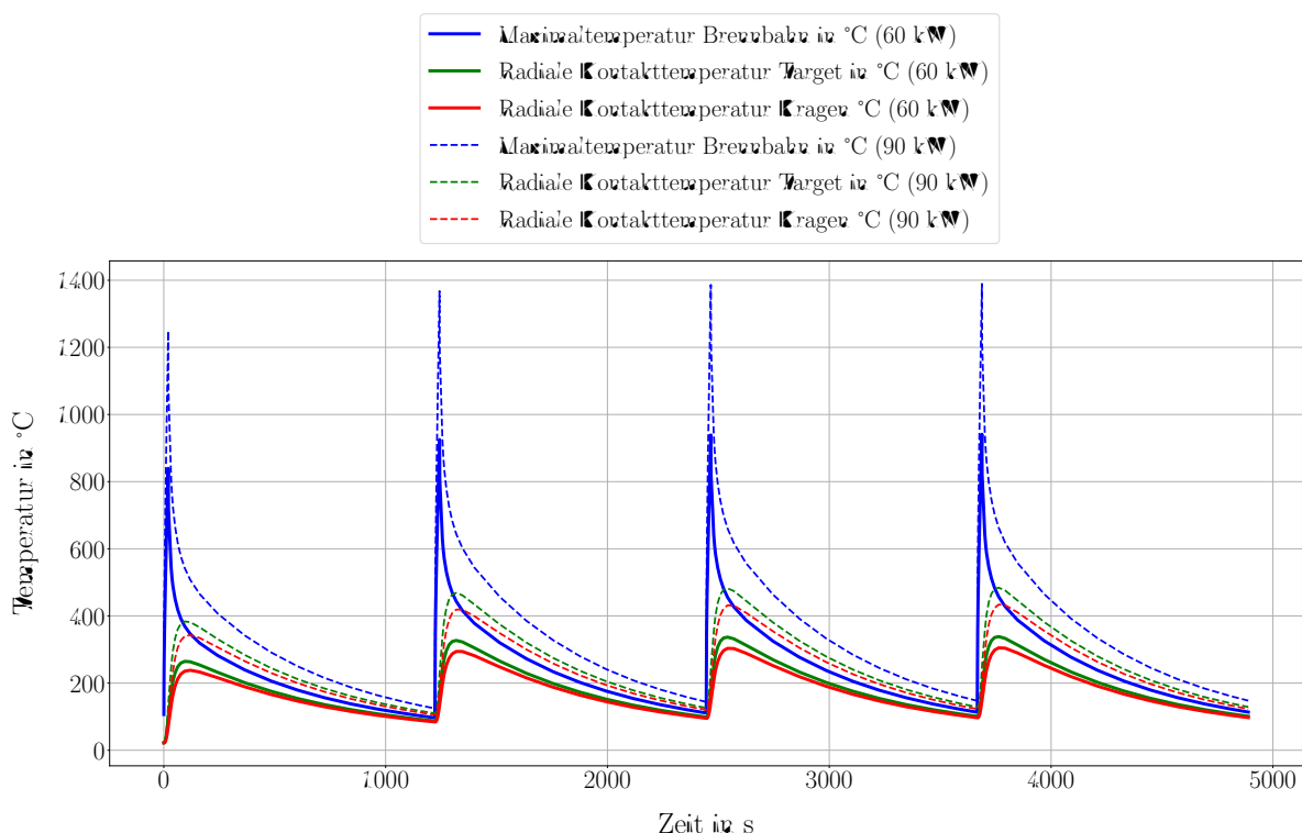
Abbildung 5.14: Temperaturgegenüberstellung für den reduzierten Lastfall von 60 kW in Gegenüberstellung mit voller Leistung (90 kW)
