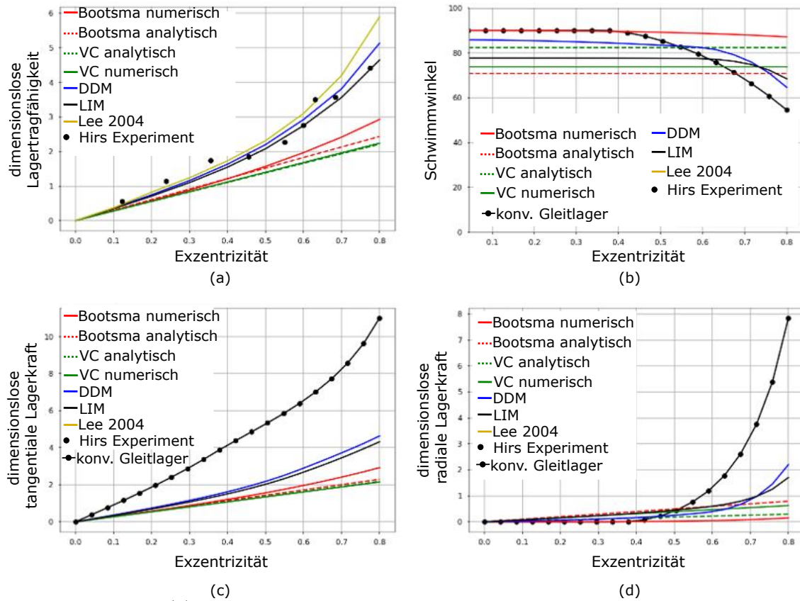
Abbildung 4.16: (a) Dimensionslose Lagertragfähigkeit mit experimentellen Daten von Hirs
