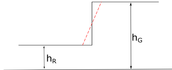
Abbildung 4.11: Modellierung der Schräge an Rille-Damm-Grenzfläche
