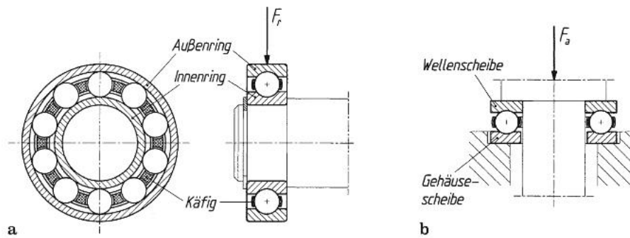
Abbildung 2.1: Aufbau eines Wälzlagers. a) Radiallager, b) Axiallager [62]
